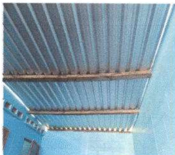
Foto 1 : sustitucion de lámina, por lámina troquelada aluzinc calibre 26 en modulo 2
